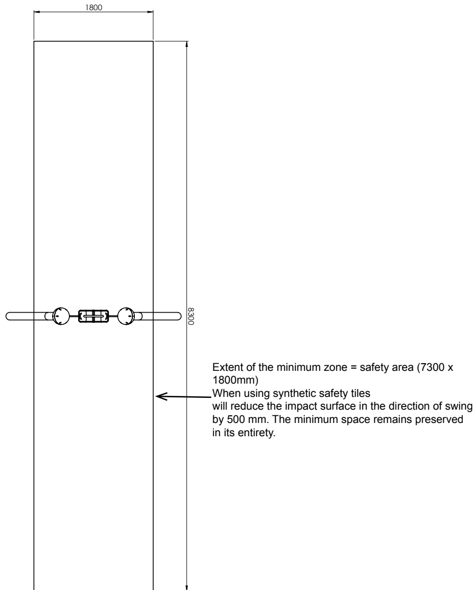
Skizze 3: Draufsicht „divo“
