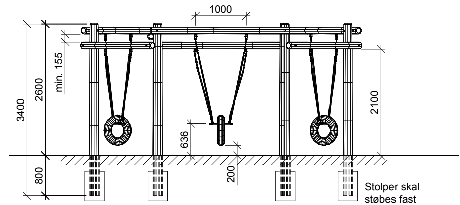
Sidebillede
