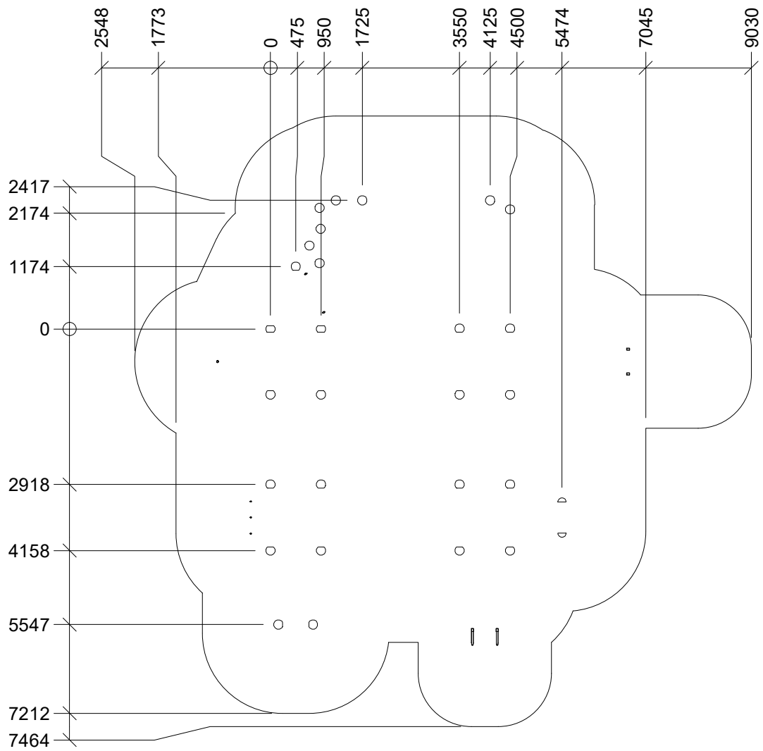
A-A (1:100)
