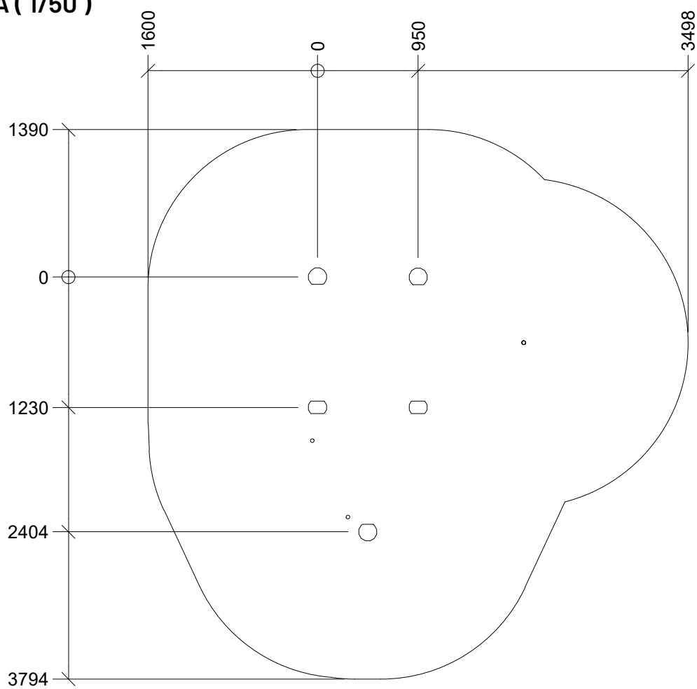
A-A ( 1/50 )
