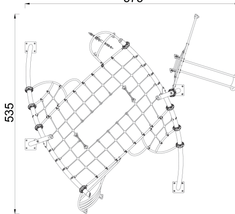
ÜST GÖRÜNÜŞ / TOP VIEW
