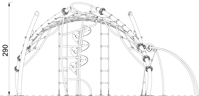
ÖN GÖRÜNÜŞ / FRONT VIEW
