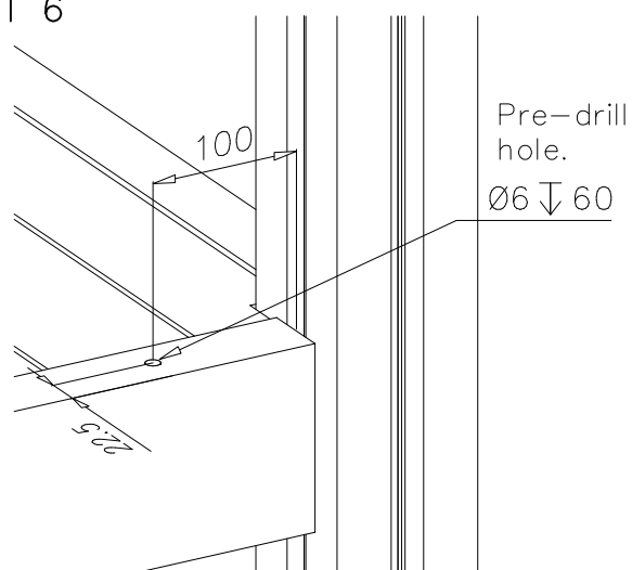
DET 6
