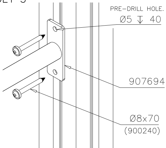
DET 5
