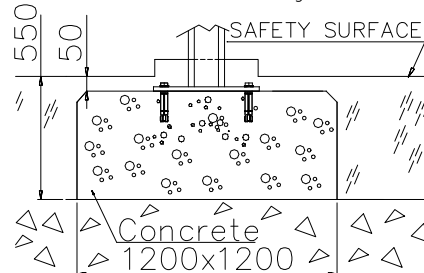
DET 36
